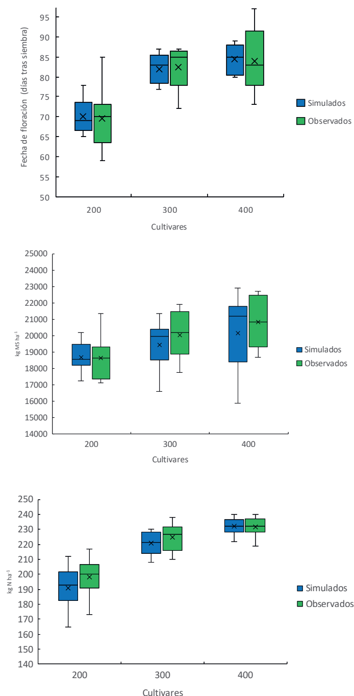
Figura 2. Diagrama de cajas y bigotes de los valores medios de la fecha de floración masculina, producción de materia seca de la parte aérea de la planta entera y producción de nitrógeno de la parte aérea de la planta entera para tres cultivares de maíz forrajero en tres localidades: Barcia, Villaviciosa y Grado, y tres años: 2012, 2013 y 2014. Simulación con limitación de agua y nitrógeno
