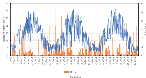
Figura 1. Datos meteorológicos observados diarios durante los años de evaluación (2012-2014) en las fincas experimentales de Barcia, Villaviciosa y Grado (Asturias)
