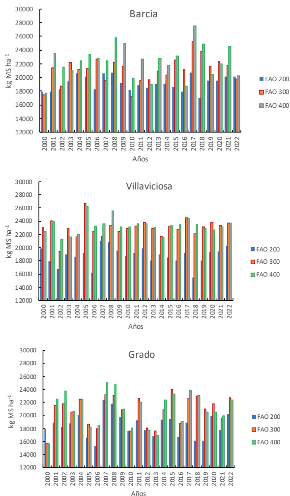
Figura 3. Comparación de la producción de materia seca de la planta entera ( \text{kg MS ha}^{-1} ) simulada mediante 23 años de datos meteorológicos en Barcia, Villaviciosa y Grado para los tres cultivares estudiados (FAO 200, FAO 300 y FAO 400)
