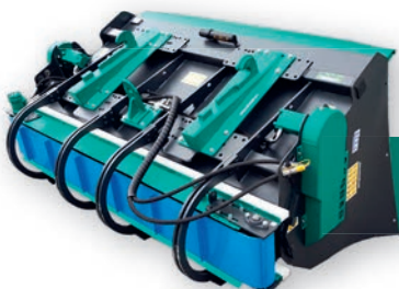
ENCAMADORA DE CUBÍCULOS ENCAMADORA DE CUBÍCULOS DE 1.7 m 3 Y 2.1 m 3
