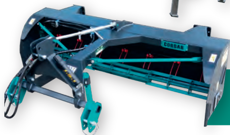
NIVELADORA AGRÍCOLA DE 3 PUNTOS
